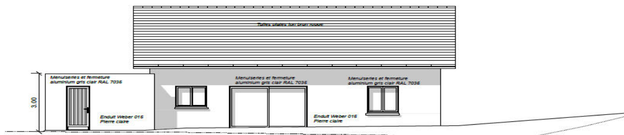
Façade Sud
