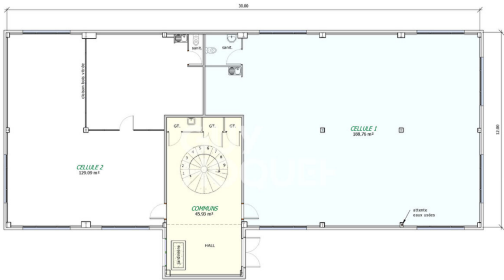
IMMEUBLE LE CENTAURE PLAN NIVEAU RDC SURFACE UTILE = 363.79 m² Echelle 1/100
